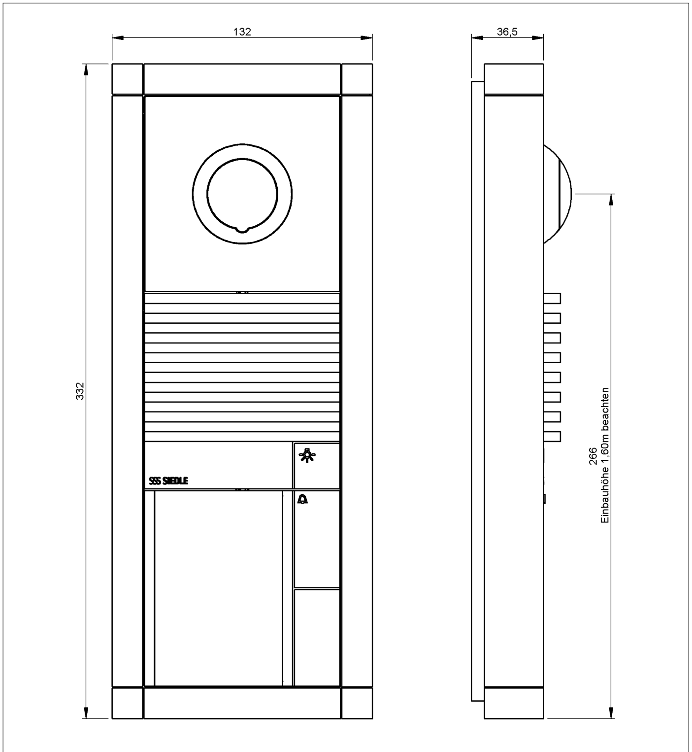
Vario Türstation: GA 612-3/1-0 Vorbereitet für den Einbau: BCM 653-02, MR 611-3/1-0, BTLM 650-04, BTM 650-01
