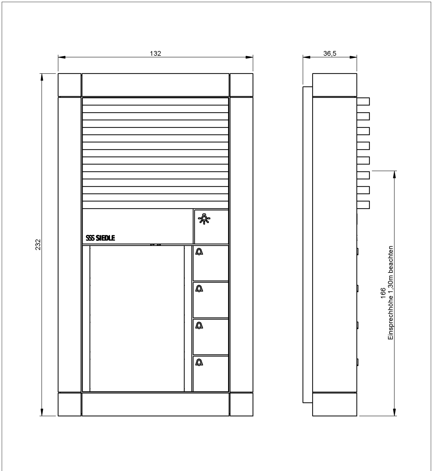
Vario-Türstation: GA 612-2/1-0 Vorbereitet für den Einbau: BTLM 650-04, MR 611-2/1-0, BTM 650-04
